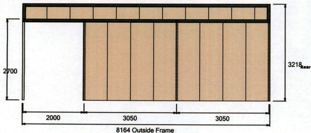
Right Elevation
