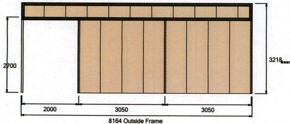
Right Elevation
